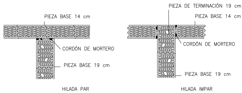
DETALLE DE ENCUENTRO EN T DE MURO DE 19 cm CON MURO DE 14 cm
