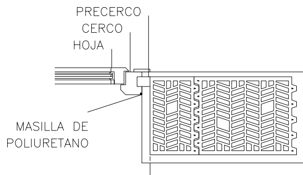
Figura 30: Jamba.
