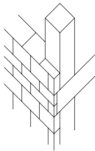
EL BORDE DEL FORJADO SOBRESALE 5 cm
