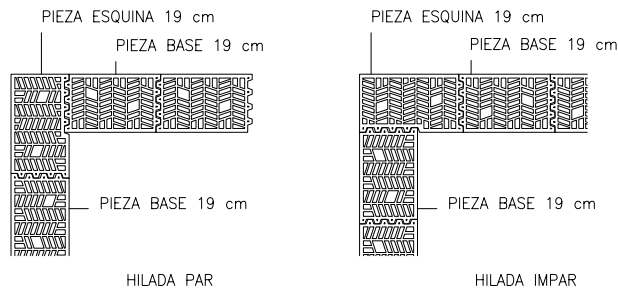
DETALLE DE ESQUINA DE MUROS DE 19 cm CON PIEZA DE ESQUINA
