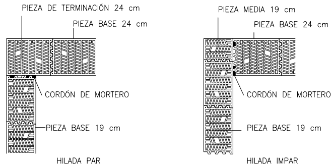
DETALLE DE ESQUINA DE MURO DE 19 cm CON MURO DE 24 cm
