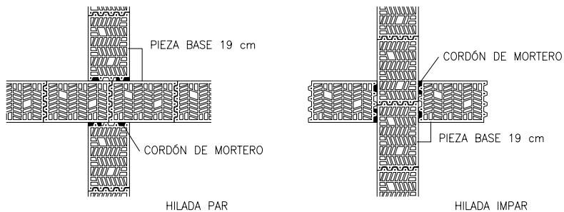
DETALLE DE CRUCE DE MUROS DE 19 cm
