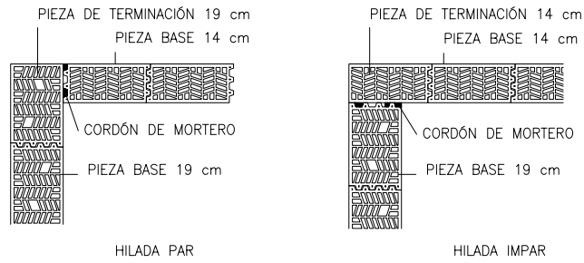
DETALLE DE ESQUINA DE MURO DE 19 cm CON MURO DE 14 cm
