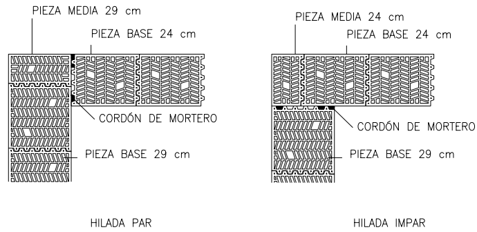
DETALLE DE ESQUINA DE MURO DE 29 cm CON MURO DE 24 cm
