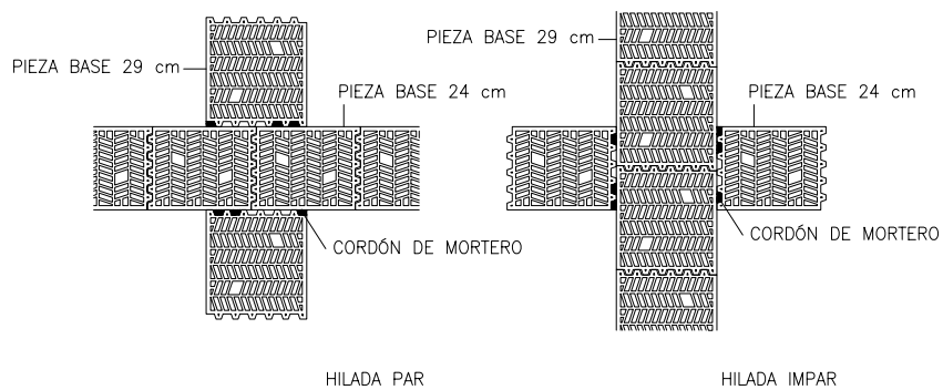
DETALLE DE CRUCE ENTRE MURO DE 29 cm Y MURO DE 24 cm
