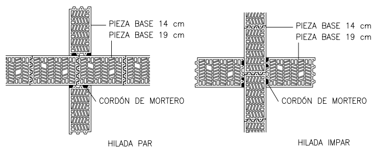
DETALLE DE CRUCE ENTRE MURO DE 14 cm Y MURO DE 19 cm
