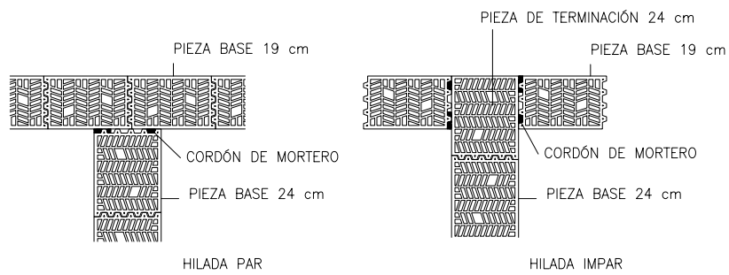
DETALLE DE ENCUENTRO EN T DE MURO DE 24 cm CON MURO DE 19 cm
