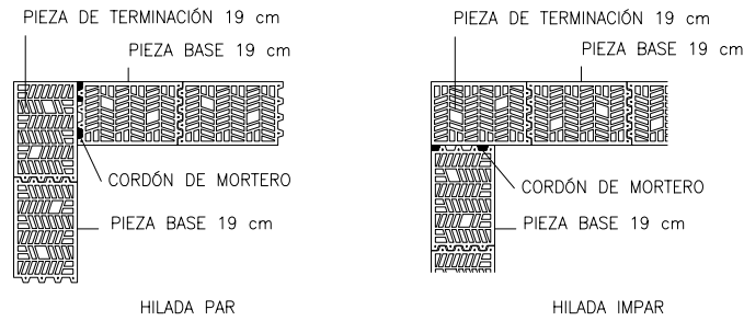
DETALLE DE ESQUINA DE MUROS DE 19 cm
