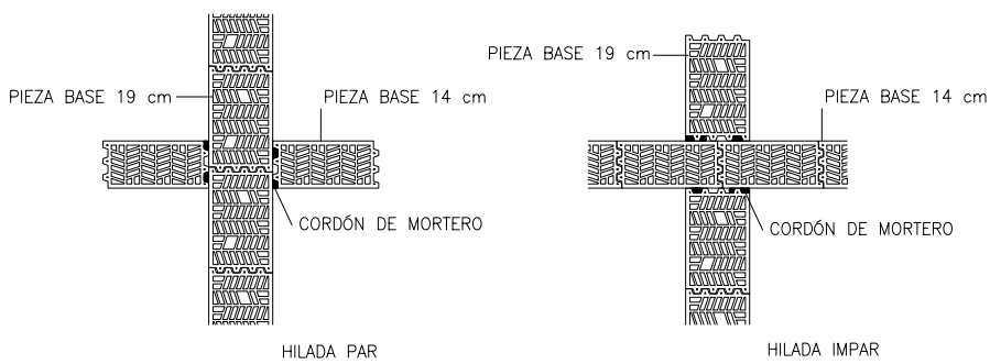
DETALLE DE CRUCE ENTRE MURO DE 19 cm Y MURO DE 14 cm
