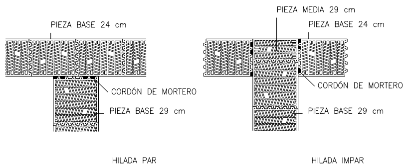
DETALLE DE ENCUESTRO EN T DE MURO DE 29 cm CON MURO DE 24 cm
