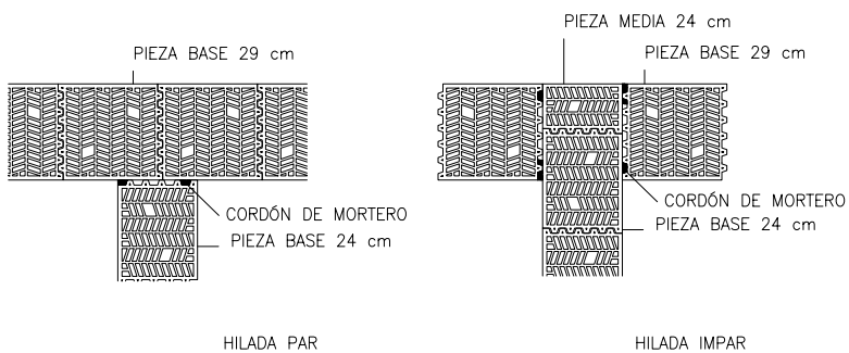
DETALLE DE ENCUENTRO EN T DE MURO DE 24 cm CON MURO DE 29 cm
